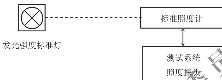
图 5 照度校准示意图
