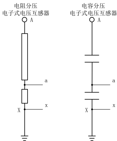
图 1 电子式电压互感器原理图
