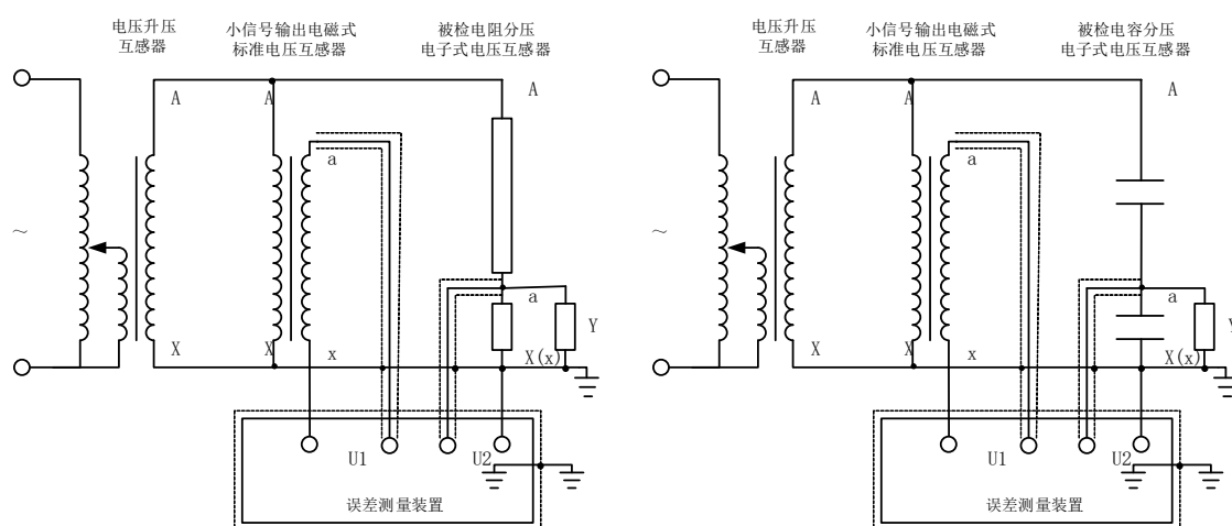
图 3 小信号输出标准电磁式电压互感器做为标准器的线路
