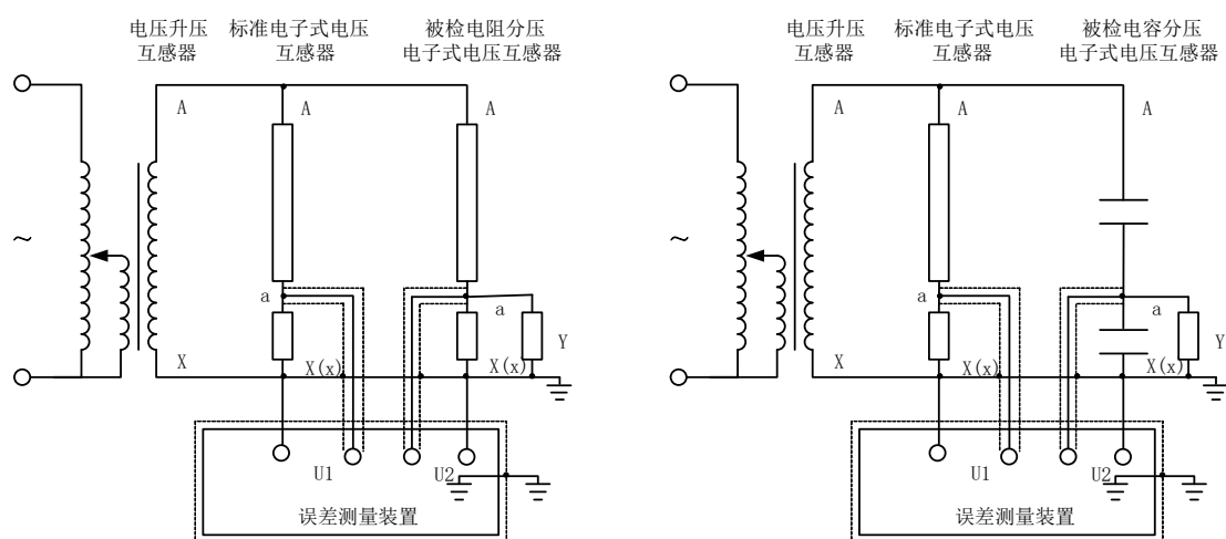
图 2 标准电子式电压互感器作为标准器的线路
