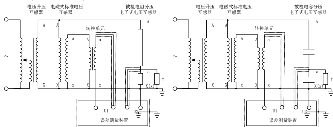
图 4 组合标准器作标准器的线路
