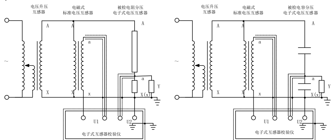
图 5 电子式互感器校验仪做误差测量装置的线路
