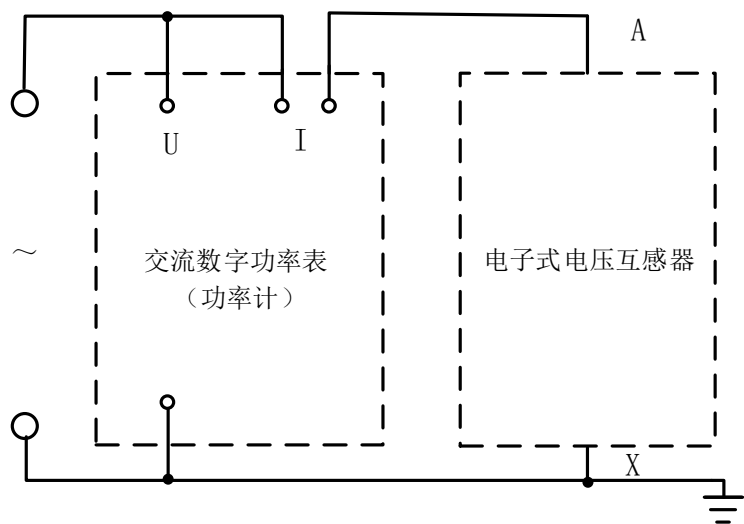
图 A.1 电子式电压互感器空载损耗测量线路
