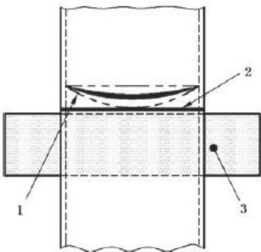
其中：1——弯液面；2——分度线或环形标志线；3——深色（蓝色或黑色）纸带
