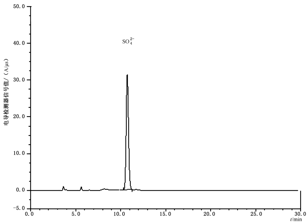
图 C.1 二氧化硫标准工作溶液( \text{SO}_4^{2-} )离子色谱图(10 μg/mL)
