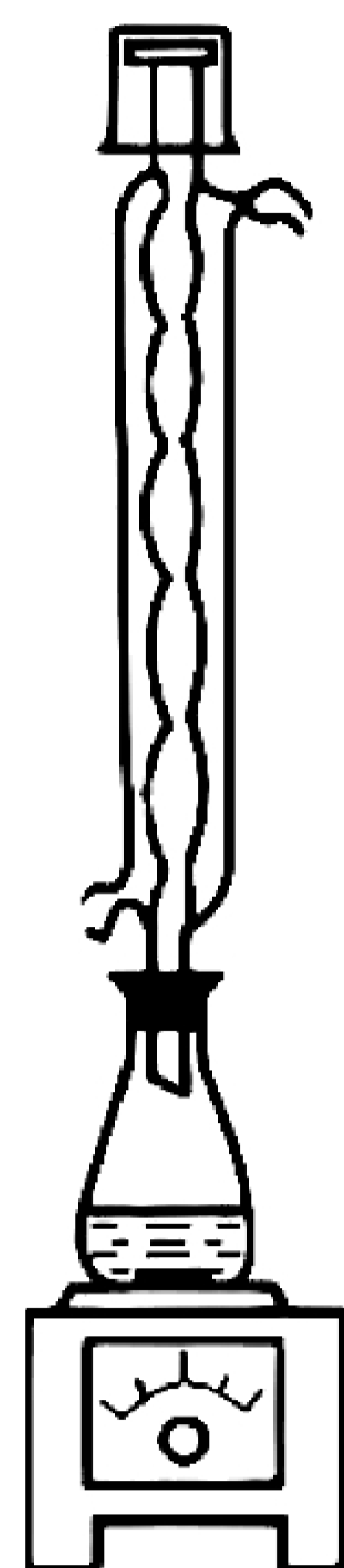
图 1 加热回流装置示意图
