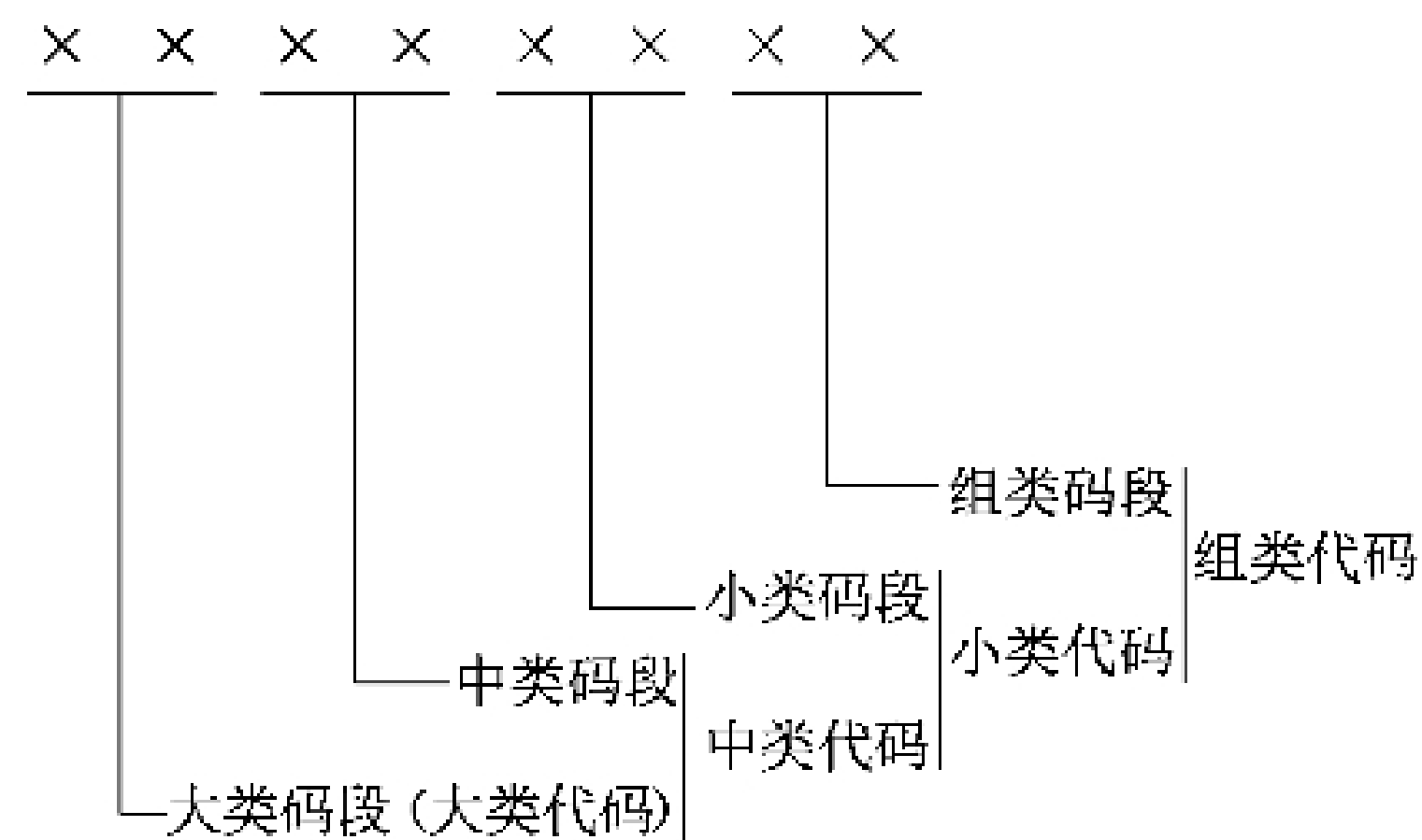
图 1 代码结构
