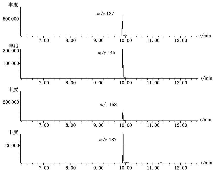
图 B.2 单辛酸甘油酯生湿面制品基质匹配标准溶液(50 μg/mL)的气相色谱-质谱选择离子监测(SIM)色谱图
