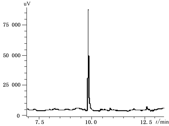
图 B.1 单辛酸甘油酯标准溶液(50 μg/mL)的气相色谱图
