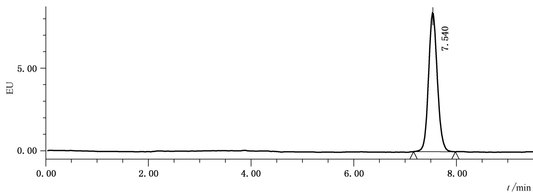
图 A.1 乙氧基喹标准溶液(20 ng/mL)的液相色谱图
