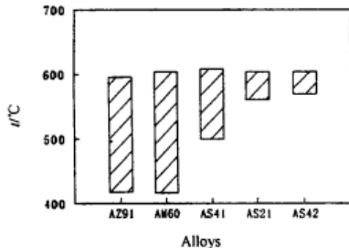
压铸镁合金的凝固温度范围
