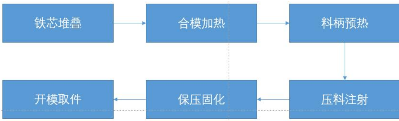
热固工艺关键步骤
