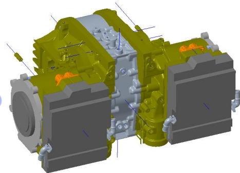
E802电驱
