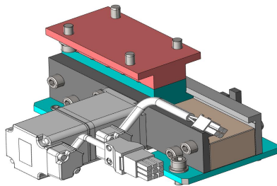
结构图
