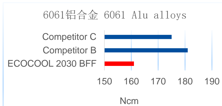
摩擦模拟/切削扭矩测试 (扭矩越低越好)
