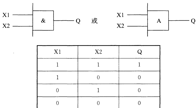
图 2~图 7 中电磁阀的逻辑应符合以上定义。
