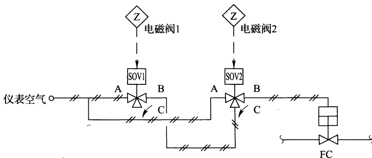
图 7 切断阀带冗余电磁阀配置示例
